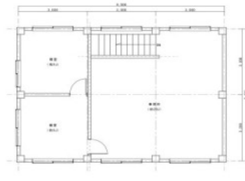
2階平面図
