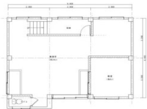
1階平面図
