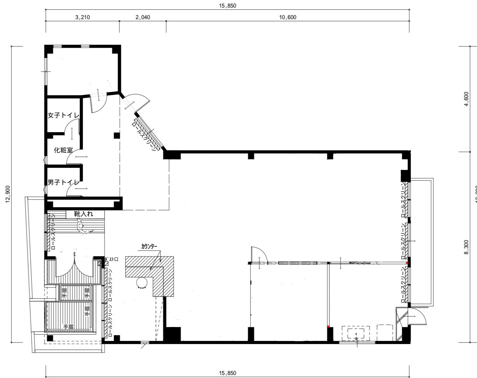
平面図 S:1/100
